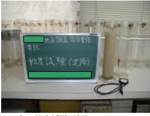
土の粒度試験(沈降)
