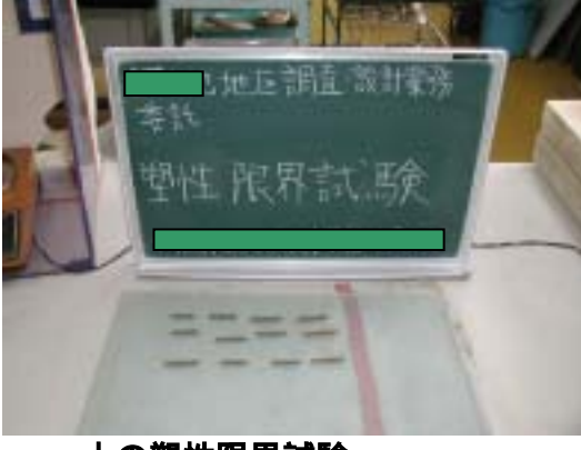
土の塑性限界試験
