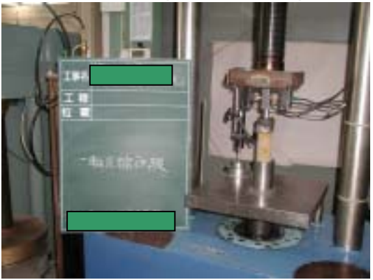
土の一軸圧縮試験
